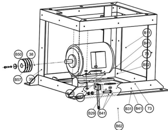
FRAME DIE ASS'Y
